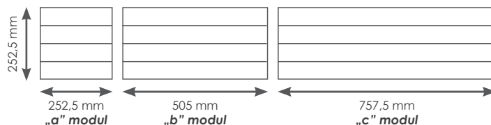
ALUTILEMAT® COMPACT 4 SÍNES MODULOK
