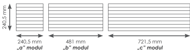
ALUTILEMAT® MINI 8 SÍNES MODULOK
